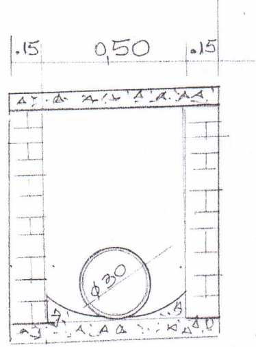
CORTE CD
