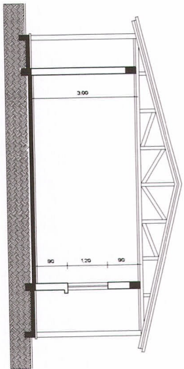
CORTE B/B' ESCALA: 1/500
